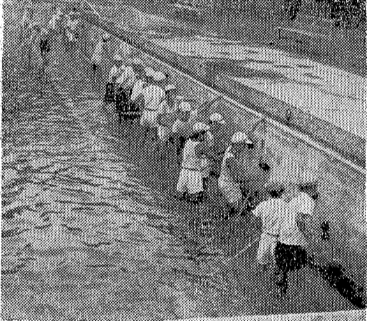
平市第三中学校の校庭拡張工事現場
