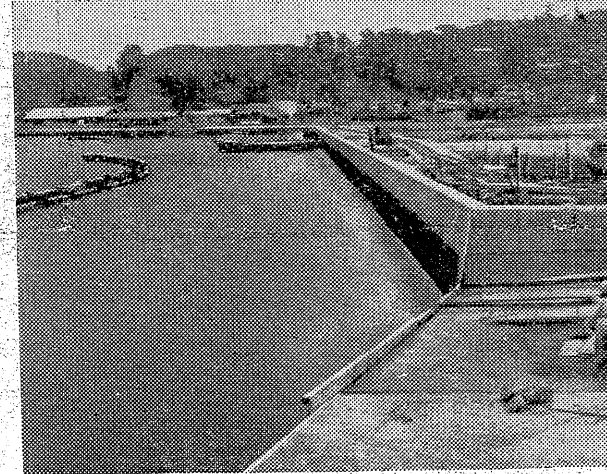
写真：完成した三噸地先の荷揚場
