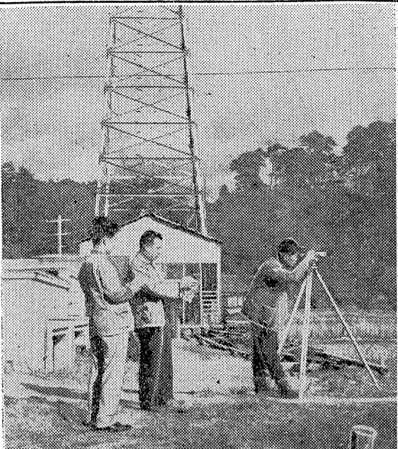
湯場ボーリング付近の実地測量 (後方のヤグラが白鳥温泉ボーリング)
