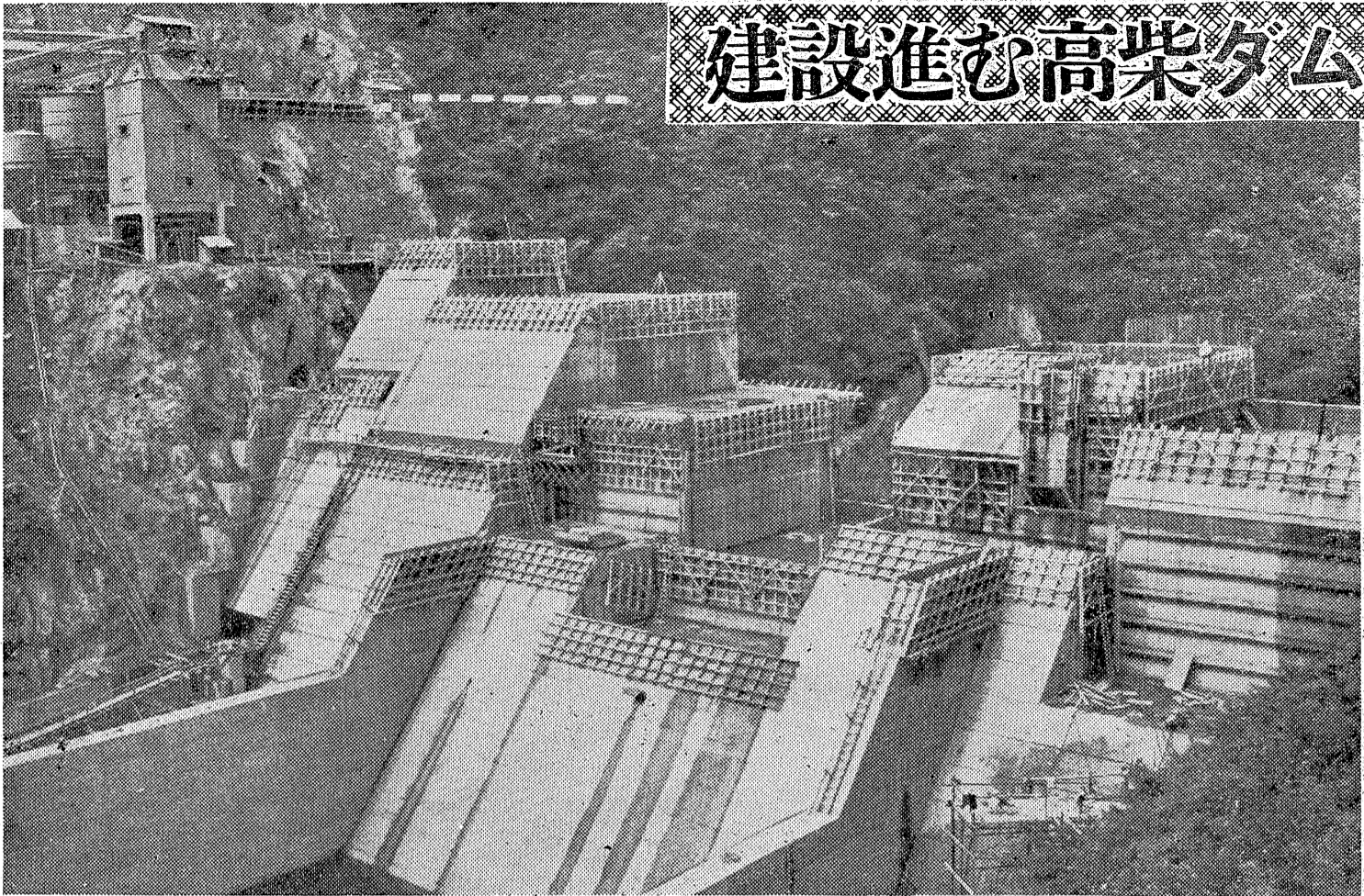
点線の位置五八分の高さまでダムが築かれ、完成すると総貯水量二千七百七十五万立方メートルの巨大なダムが出現する
