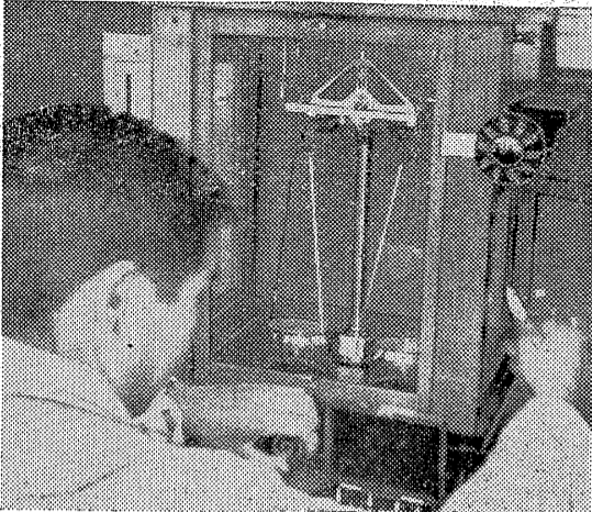
ハカリは正確さが大事だが、化学分析用には百分の一ミリ以下の単位が必要となってくる。計量する場合、風圧・水平・温度など厳密な注意のもとに、器具に手をふれずピンセットを用いてはかる。写真は硝子箱に収めたまま計量する平工の化学精密天びンバカリ。
