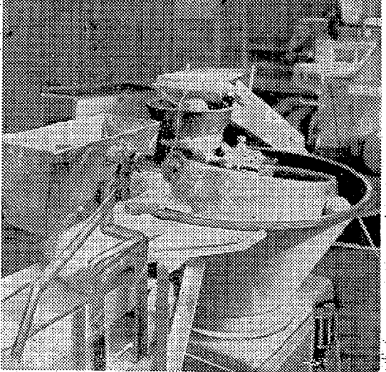
小麦粉を適度に練り混ぜる自動混合機
