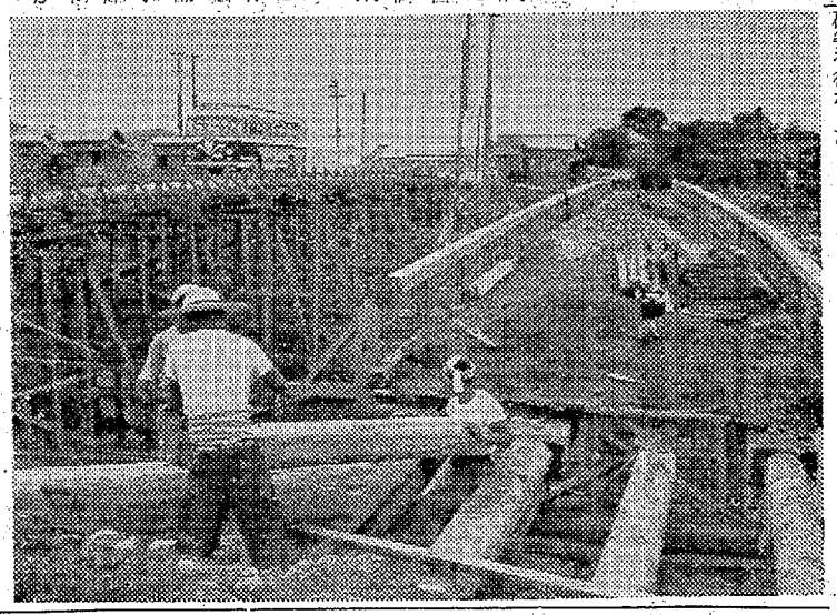
【平川橋の架け替え工事で板橋が架け置かれた。】
