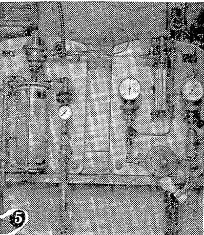
④必要量に応じてバルブの開閉で水量を調整し⑤濾過して滅菌消毒して平市八幡小路の配水池に二本のパイプで送水する
