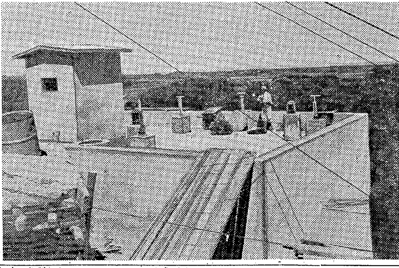
草野地区簡易水道第二期工事の建設現場。配水池とポンプ場の基礎が完成している。
