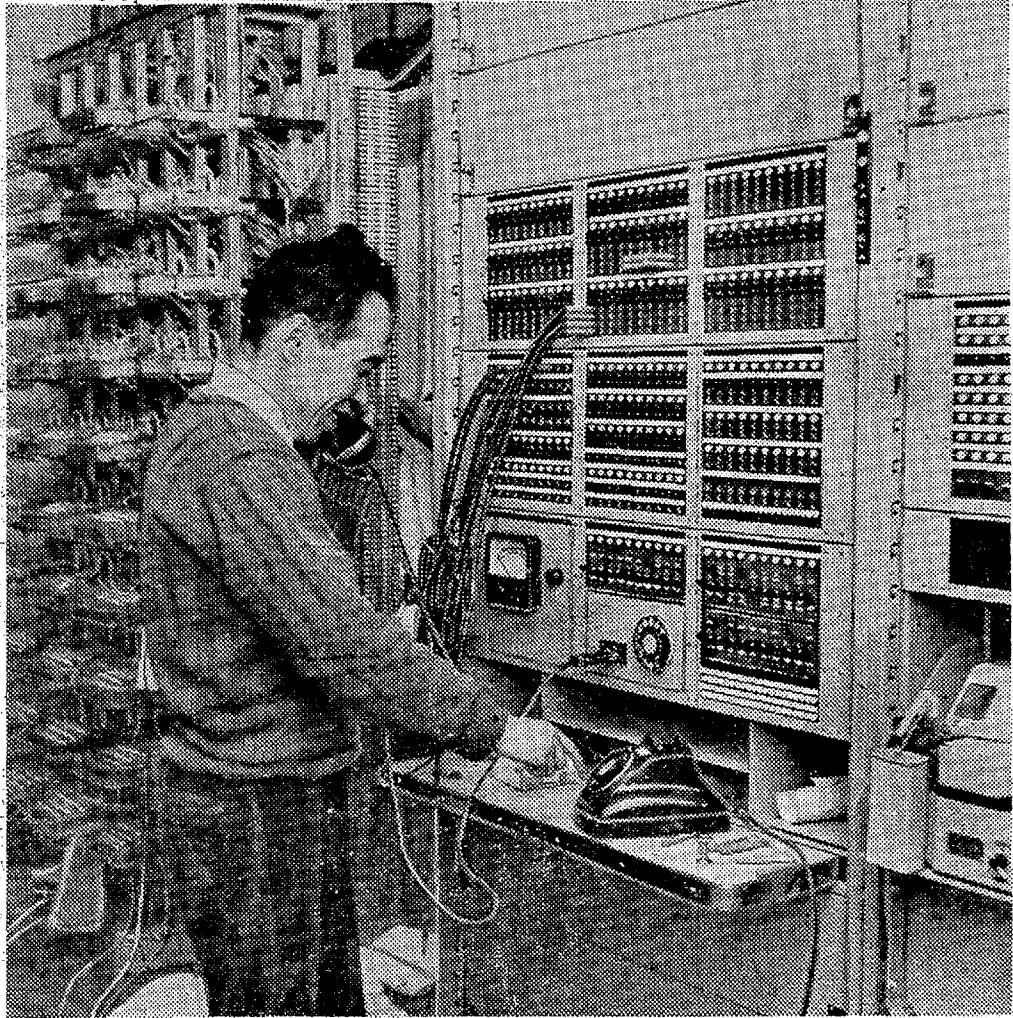
ダイヤルを回して通話の試験
