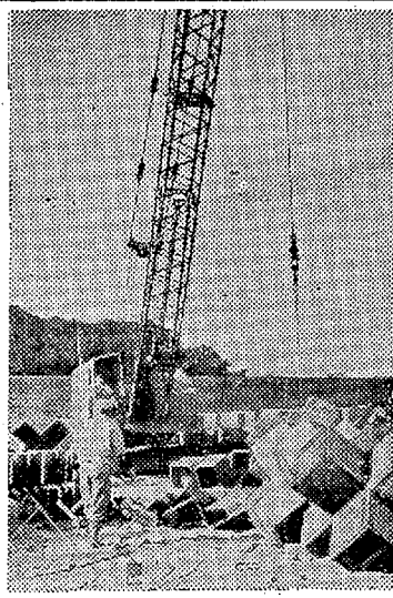
防潮堤の築設は水位約三層を掘ってコンクリート被覆型、高さ約二層の高さを保つて、防波と防潮堤の根柢を確保して六脚ブロック(重量二・三トン)を造って、鉄線網で二層に並列し、高潮に備える仕組みとなっている。
