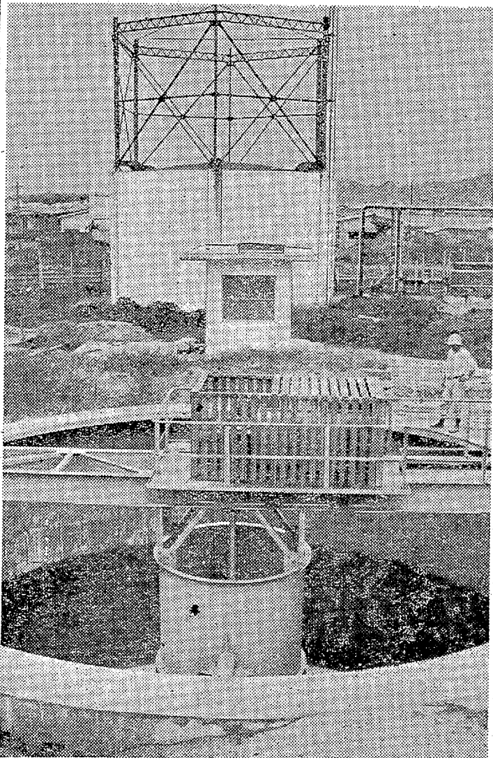
手前から沈でん槽 滅菌室発生したガスを収めるガスタンク ガスは 還元して終末処理場に使用する合理的な仕組みだ
