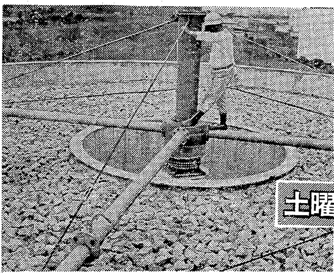
とがった砕石がぎっしり敷きつ められている高速ろ床の内部
