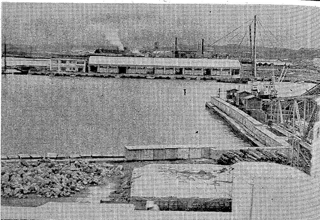
ほぼ完成した2号ふ頭 手前右側は石炭専用ふ頭=1号ふ頭のノルウェー貨物船ハマール号(12・6・92トン)船上から望む
