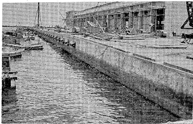
2号ふ頭の岸壁は長さ195m水深9m、1万トン級2隻が案に横付けになる
