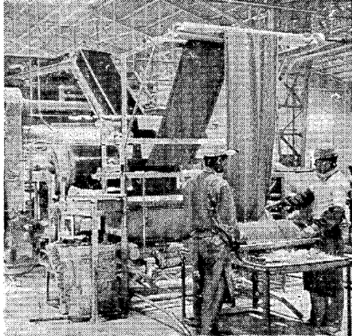
【生地出し逆しカレンダーロール】同社研究新作の秘密兵器 ゴムが織り物のように出てくる
