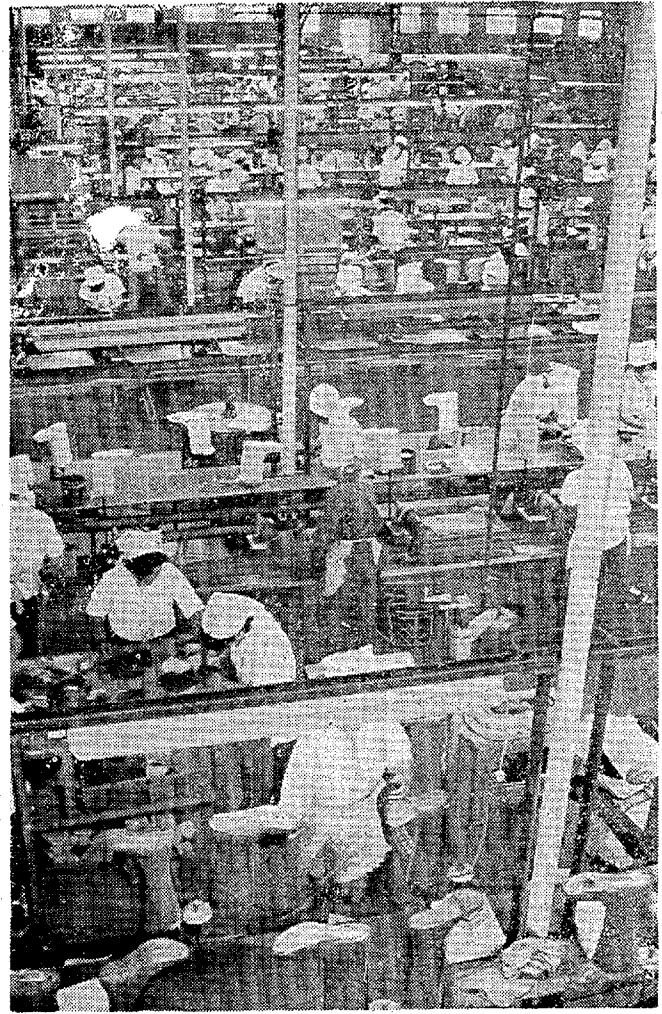
【ジャッキコンベア】全部で9台 1台17工程 裏布をかぶせ ひと回りするとゴム長ができる
