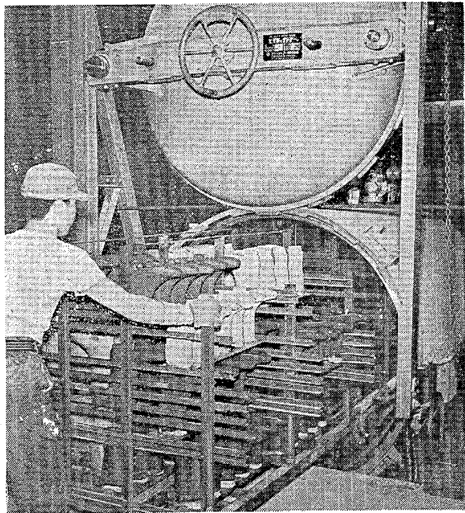
【加硫機】カマである はり合わせたゴム長にツヤ出し塗料 一時間で焼きつける最後の工程
