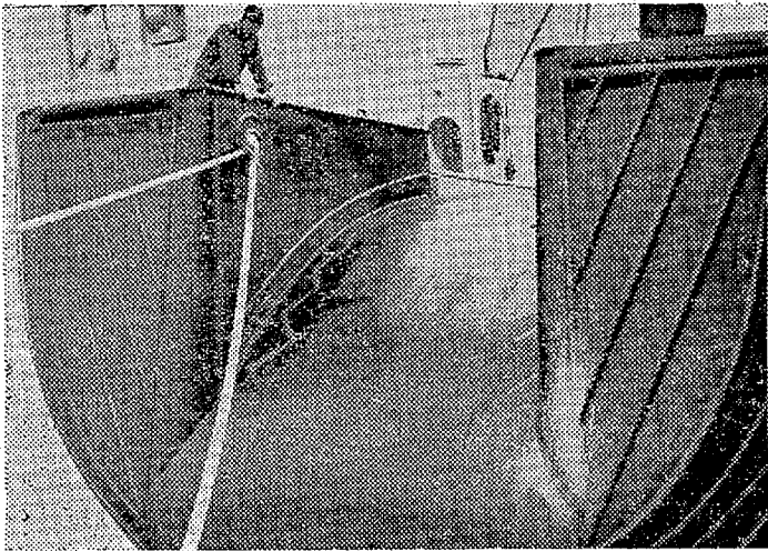
船尾式トロール船の漁網の引き揚げはこの凹型船尾を利用する合理的なもの
