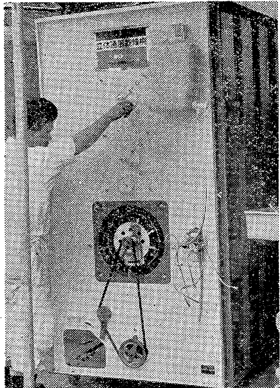
刈り入れた稲 ムギなどの穀類を1度に80%乾燥する分解組立式の立体通風乾燥機
