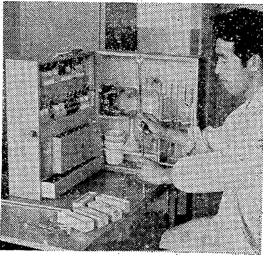
携帯用の現場水質分析器、このほか常置のものもある
