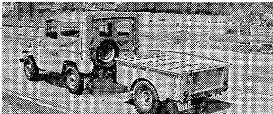
化学薬品「ドライケミカル」20リットル29本を積める補給車
