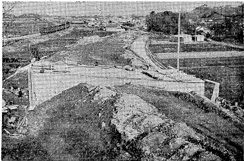
土盛りもほぼおわり。橋脚工事に入った鎌田谷地内の新設の取付け道路。
