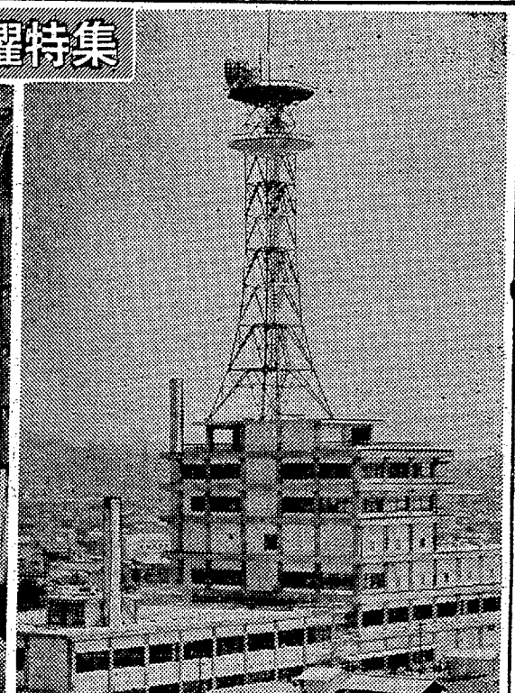
近代通信科学の粋が秘められている平電報電話局全景 パラボラは神楽山と向かい合っている
