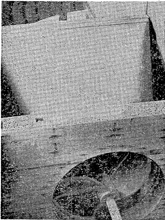
回流水槽はプロペラを回転させ 水流を自在に変化することができる 海流がそのまま再現する
