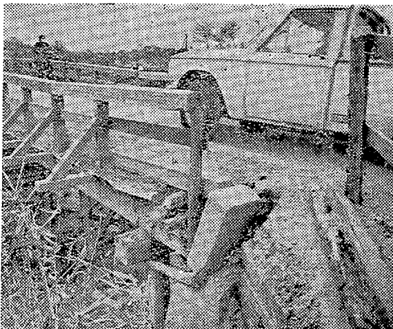
橋のいたみはひどい 新橋と合わせて早急な補修工事が望まれている
