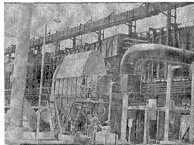
除塵装置ロートクロン
