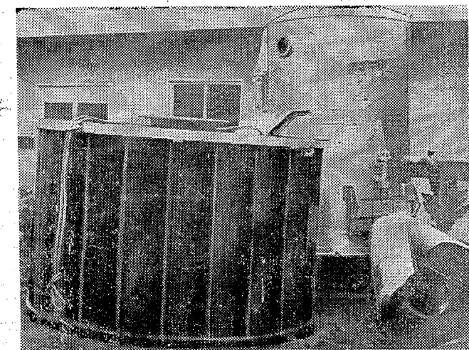
防熱用の冷海水貯蔵タンク(手前)と真空式フィッシュ・リフター
