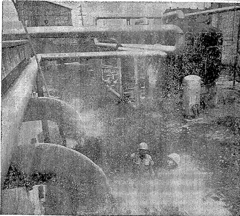
毎時百トンの能力の過熱器が二重設置され、熱湯の蒸気は、経済省省ないコンクリート製の貯湯槽に送られる。
