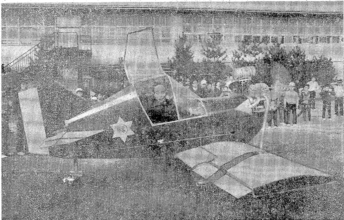
地上滑走機 E I 1号 翼長3.6m 機長3.2m 250CC 22馬力 1人乗り 飛行機と同じ設計で、わがと飛ばないようにした プロペラはケヤキ エンジンには中古バイクの廃物利用で工作日数は1カ月 1万5千円の費用で完成 稼働するのが中野先生
