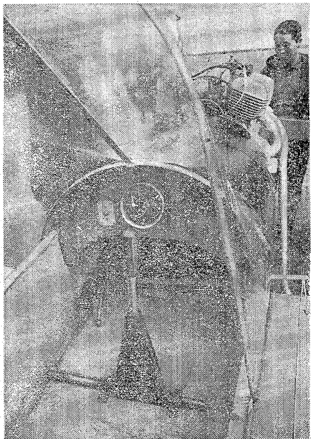
操縦席 一般軽飛行機と同じで簡易さが取りえ 計器とアクセルレバー クラッチはバイク部品の流用 操縦性能は軽くてグーである
