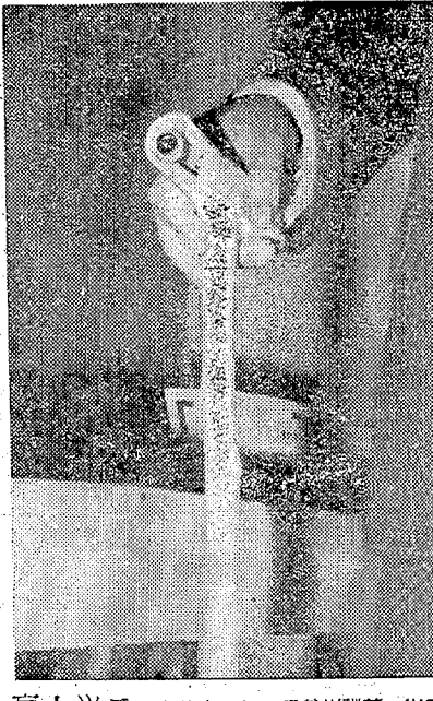
盲人ツエ 赤井中三年 長谷川訓義 ツエの先に電球と電池を入れ、スプリングとゴムの接点でツエの先が接地すると電球が点いて盲人の所在を知らせる。
