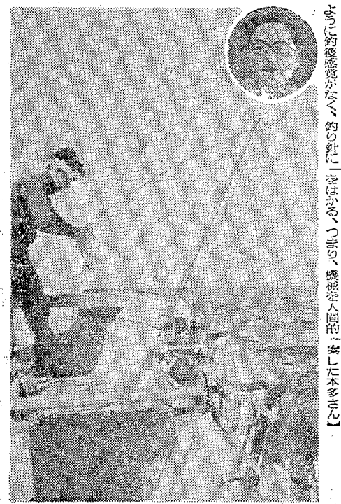
本多氏の試作した自動釣機。釣れたらブザーが鳴り、釣った魚は自動的に釣り上げられる。
