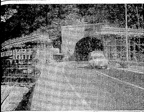
【平野町小浜町、波立遊歩道の工事現場。二トンネルと横断歩道橋の工事を行っている。
