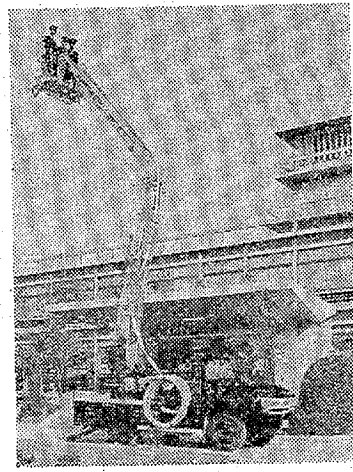
五月十三日、大阪でこの屈折式ハシゴ車と消防ポンプの試運転が行われた。この車は、従来のハシゴ車と異なり、屈折式で、消防ポンプと一体化している。
