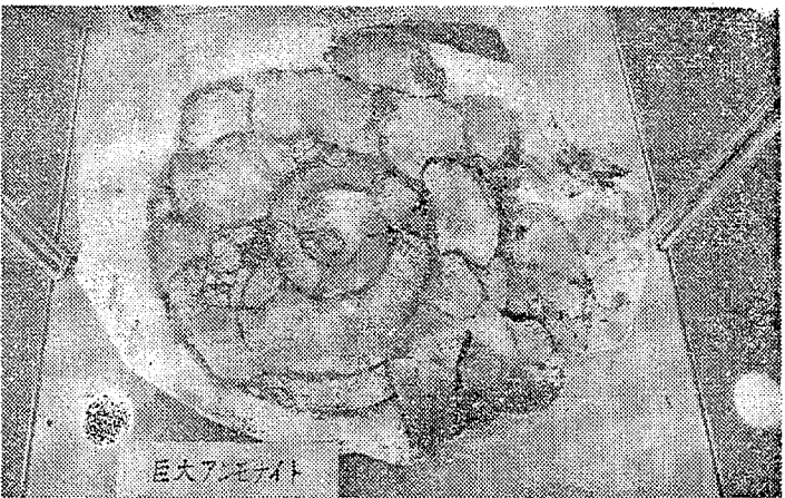
巨大アンモナイト 約8千5百万年前に生存し、現生のオウムガイと共通点が多く軟体動物に属すると考えられ、直径67センチの大久川流域で発見した化石で最大のもの。
