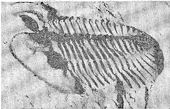
三葉虫 約2億5千万年前の節足動物で、古代の各地質時代から特有の種類が見られるので、標準化石として重要。この化石は、四倉町高倉山で発見したもので完全な形態を保っている。
