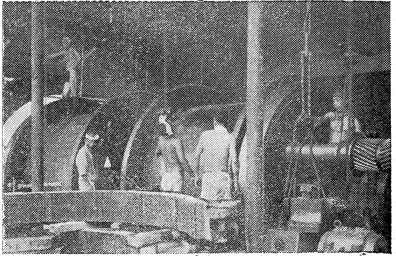
日本一の捲揚機 鹿島は一番間見ないトクコトくほどに変わる。八丁ノ巻揚場の工事に伴って抗外設備が次々とできるからである。いま組立中の千五百馬力の捲上機もその一つである。すでに機は完成して運転を開始しているが、いま組立中のものは一月から運転の予定である。斜坑捲で千五百馬力は全国でも盛城だけ、しかも二機並んで運転するようになれば偉観である。それだけ鹿島は捲揚機がかけられているともいえず、不覚に誇りにあふれる。左写真には鹿島坑の捲揚機。
