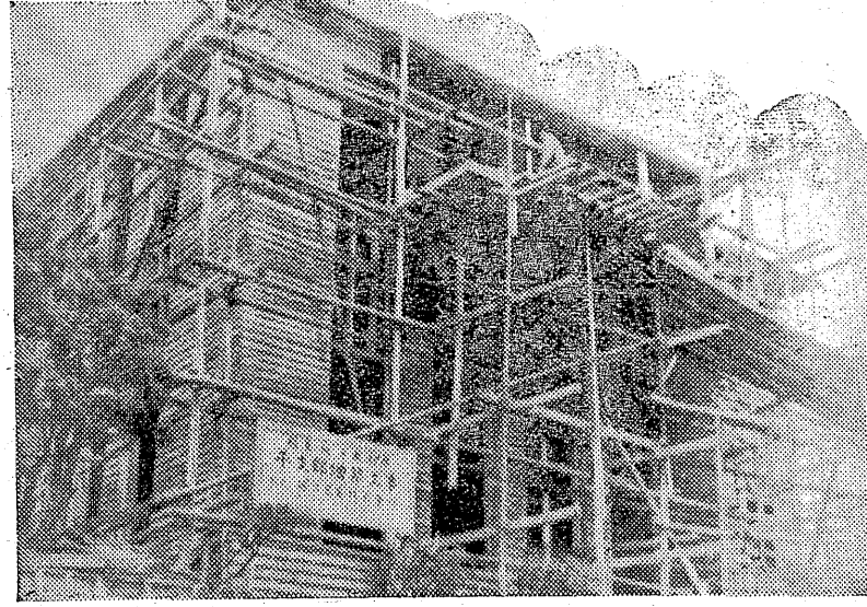
新廳舎三三三坪の敷地に總工費六百万円、堀江工業株式會社請負で三月下旬から新廳舎建造を急いで居るが七月中旬頃までに略々竣工移轉することになった、新廳舎は二階建てとなつて居り一階は支部法廷簡裁法廷に、二階は裁判官室、書記官室、會務室、書記官室、調停室と大廣間、延室の五室となつて居り、一階の天井は總防音装置が施されて法廷は被告人控室があり大シャッターを装備し、ろう下は全部木レンガの組合せで釘一本も使用せず床面には全部リノレーンを敷くことになつて居る、規模設備其の他の点で東北一を誇る廳舎が出来上る譯であり舊式なお役所型は全く八幡小路の高台に新舊容を備えて居るのを見るからにスマートである
