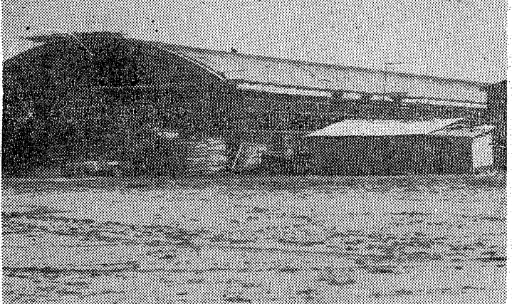
小名浜港第二、二万トン岸壁の一号上屋三万三千方メートルと管理塔六百平方メートルは総工費一億三千万円で工事を進めていたが六月中には完成する。
