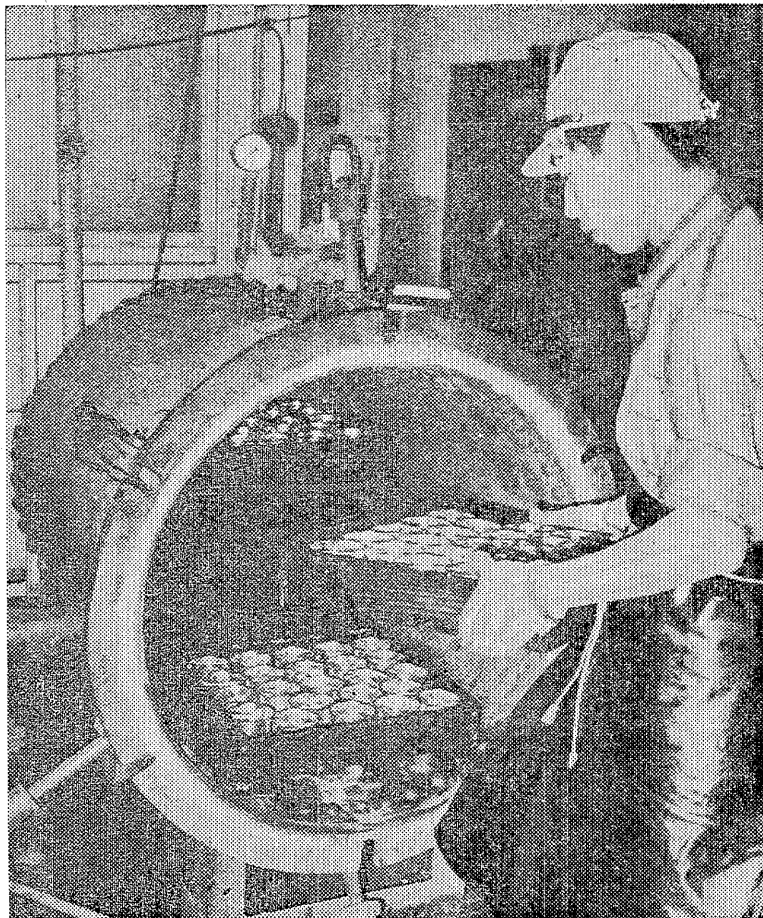
蒸気加圧釜 サンマを詰めた「カン」を入れ 高圧蒸気で煮沸と殺菌をする
