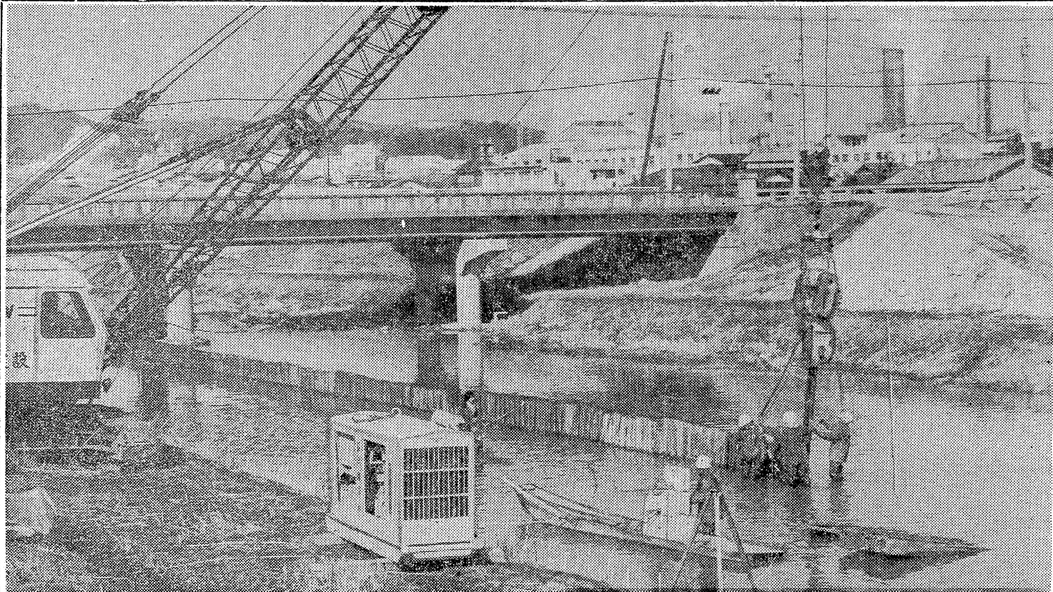
シートパイル打ち しゅんせつ作業で有害物質が海へ流れ込まないよう 川を締め切る工事が急ピッチ
