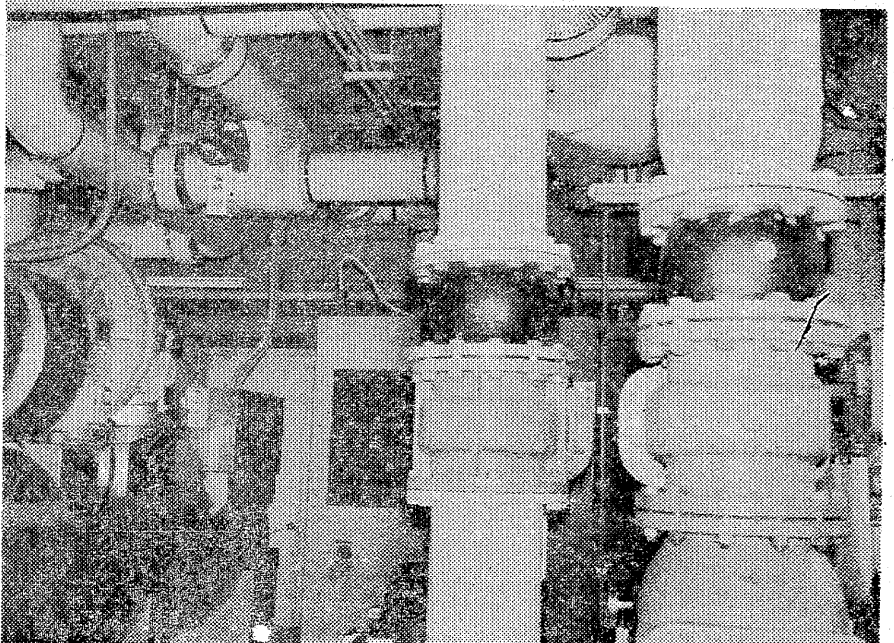
平ステーションビルの冷暖房空調設備
