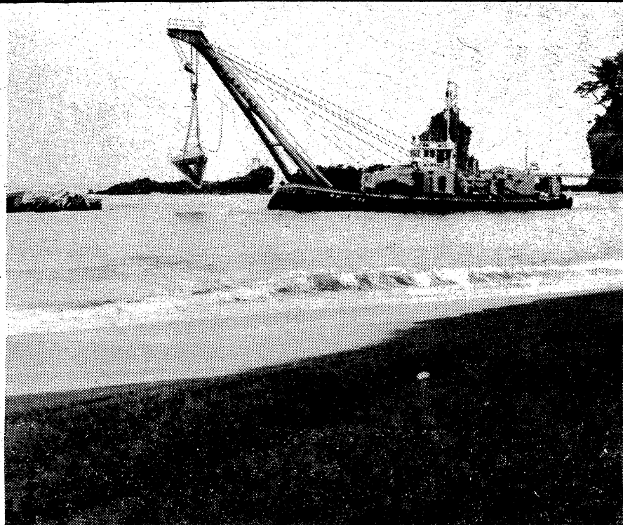
海浜を呼び戻す離岸堤作業—波立海岸
