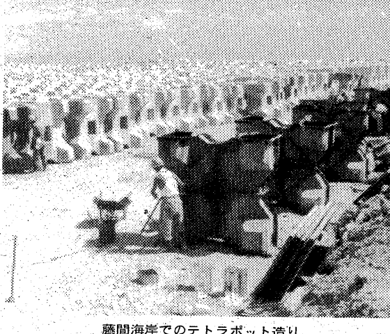
藤間海岸でのテトラポット造り
