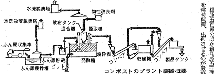
コンポストのプラント装置概要
