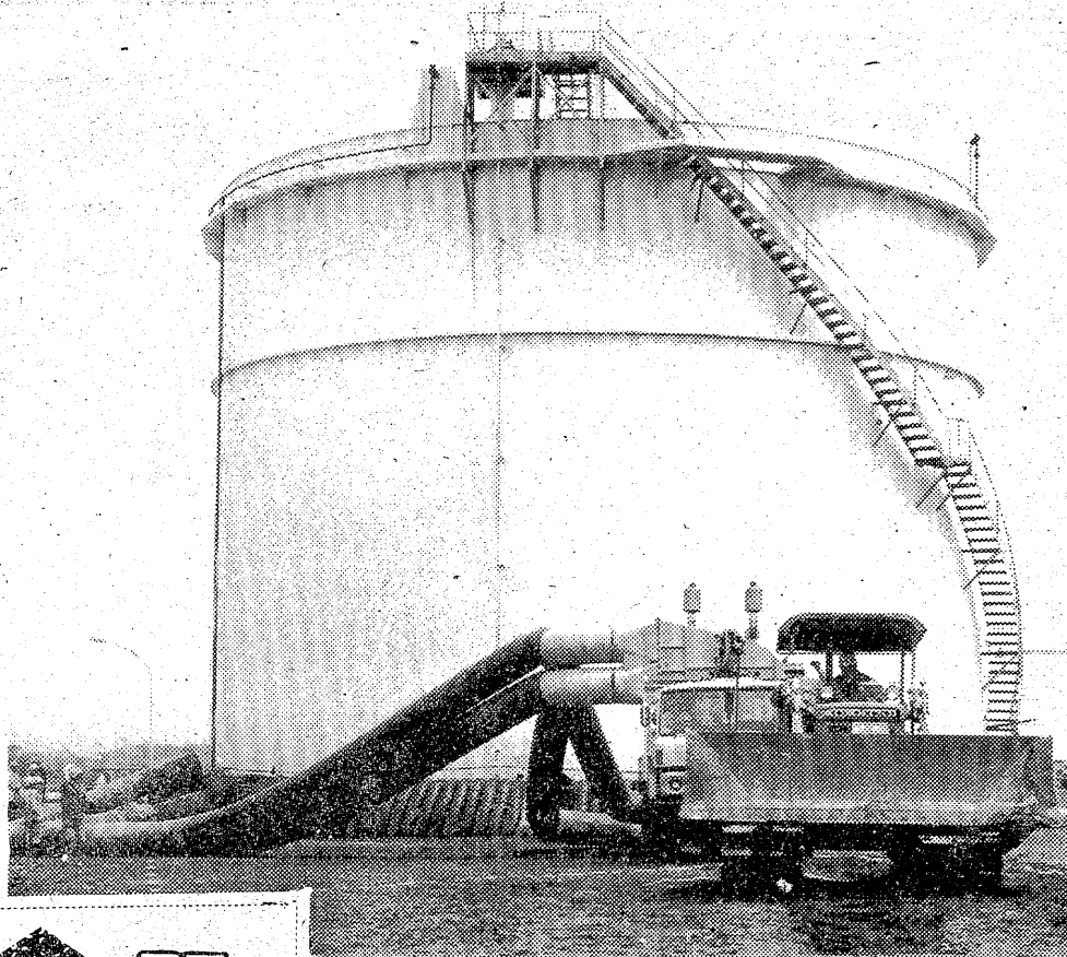
▲地盤が軟弱で将来沈下の恐れがあると富士興産小名浜石油槽所では26日から、石油タンクの移設作業を開始した。工法はイギリスが開発したエアクション法で、タンクの周囲にスカートを設置。けん引車のブローから空気を送り、スカートから噴射させ、タンクを浮かせて車で引っぱって移動させる国内初の工法は見事に成功した。
