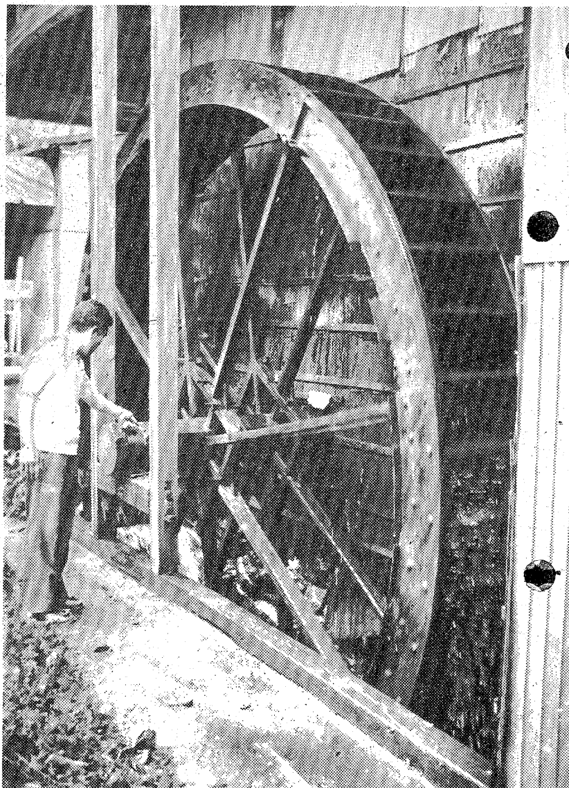
▲水車は直径が4米余 スギとカヤ、薄鉄板製でシャフトはカヤの木製 急流を利用して回転させる流水式だ
