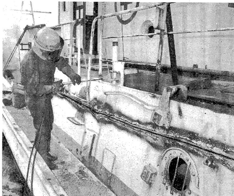
▲アセチレンガス切断機で 船橋・船首・舷側・船体の順に解 体していく 約二週間くらいで一隻がスクラップにされる
