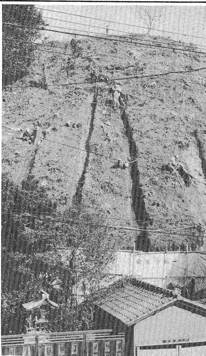
お城山(杉平地内)の急傾斜崩壊防止工事
