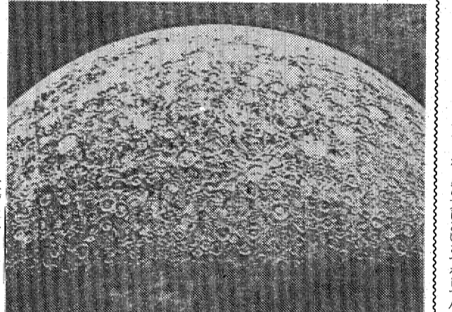
無数のクレーターにおおわれた水星の表面
