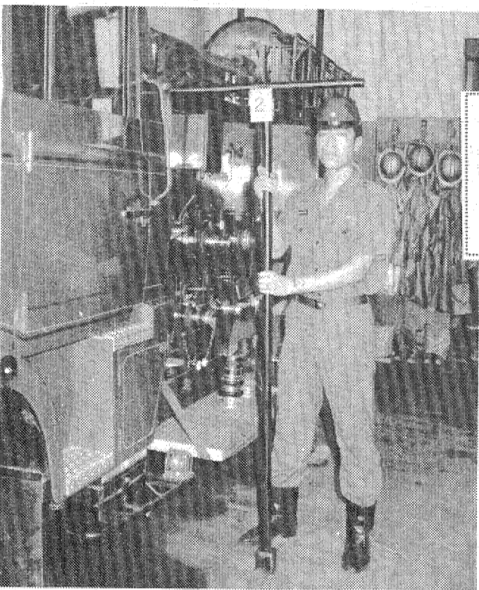
▲ガス爆発による大事故を抑止のため市消防本部は7月中旬、市内各ガス事業所と個別に、消防機関によるガスシャ断を盛り込んだ保安対策申し合わせ事項を締結した。平消防署は市内5署のトップを切って東部ガスと調印、同事業所から配管図とバルブ開閉器(写真)が渡された。同署では同器をポンプ車に常備、緊急時に当たるといふ。
