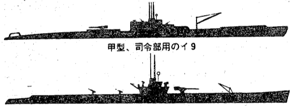
奇襲部隊揚陸用として建造されたイ361
