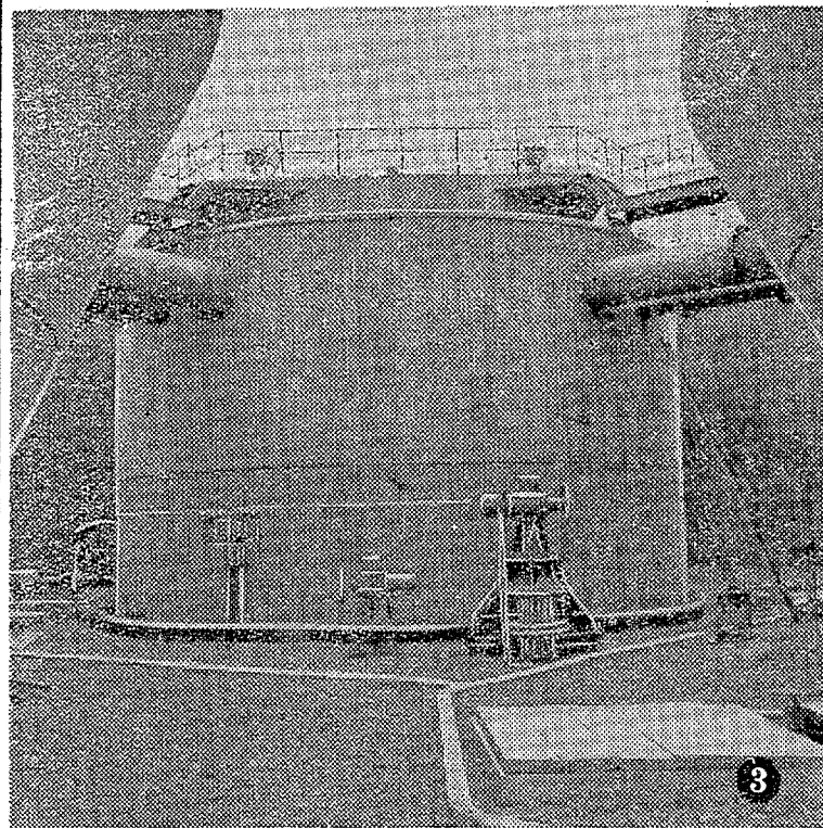
ろ水井から急速かくはん器に入り 硫酸ばん土 硝石灰を投入しかきまぜる
