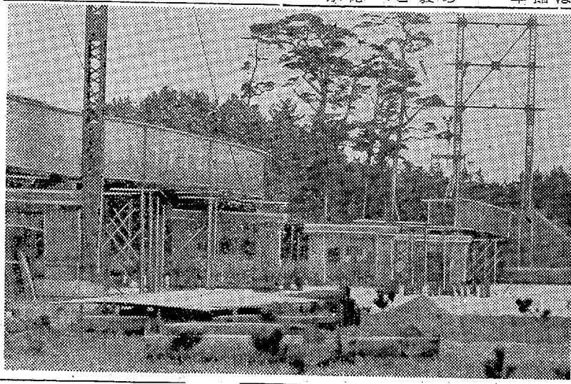
【大わたわの新舞子橋架設作業】
