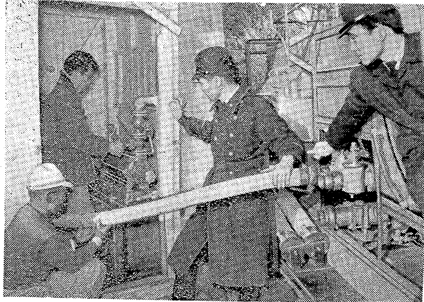
タンク車から汲れた井戸へ給水 動力ポンプで真上の灯台へ揚水する
